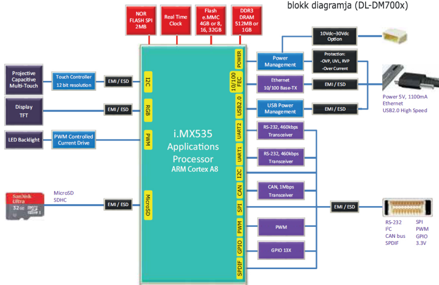
Smart Display Modul „x” sorozat blokk diagramja (DL-DM700x)
